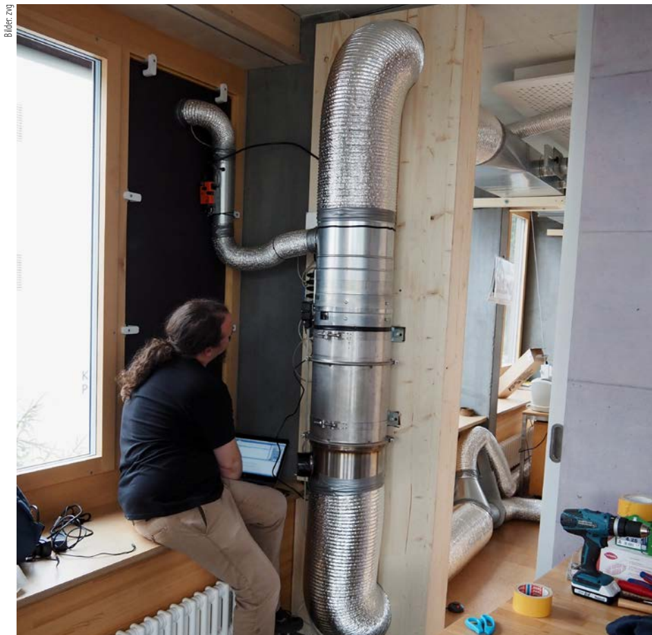
Um Lärmmissionen möglichst zu vermeiden, befindet sich das Filtergebläse in einem Nebenraum. Es erzeugt den Luftstrom im Lüftungssystem.
