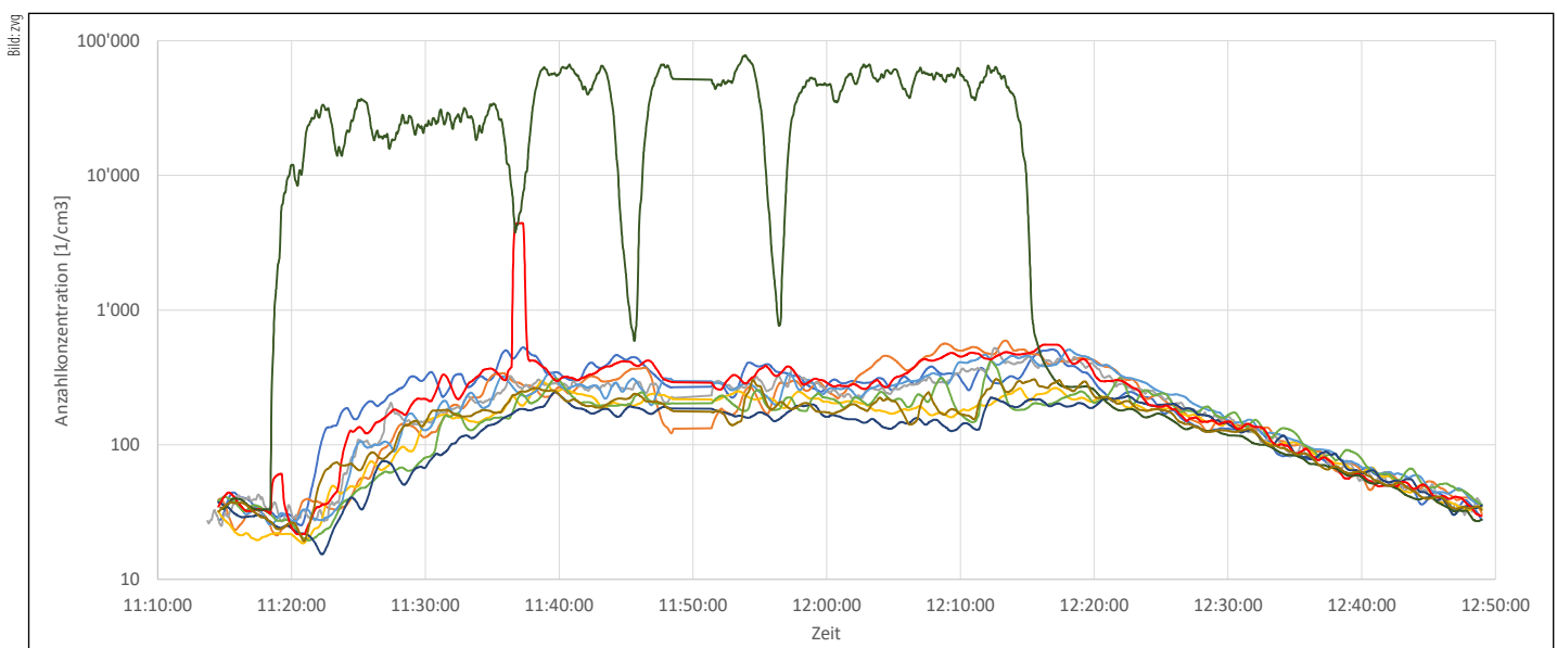
Das Diagramm zeigt die Konzentration beim Nebulizer (grüne Kurve) und an den einzelnen Pulen (andere Farben). Um 11 Uhr 20 wird der Nebulizer jeweils ein- und um 12 Uhr 15 ausgeschaltet. Die Konzentration an den Pulen ist mehr als 100 Mal kleiner als an der Quelle und im Raum überall in etwa gleich.
